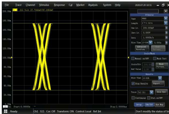
Add Jitter
