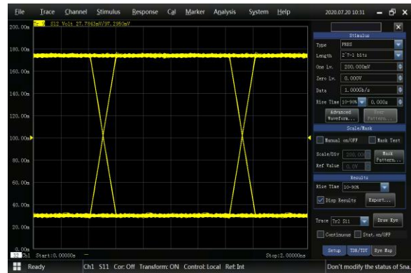
Add Noise
