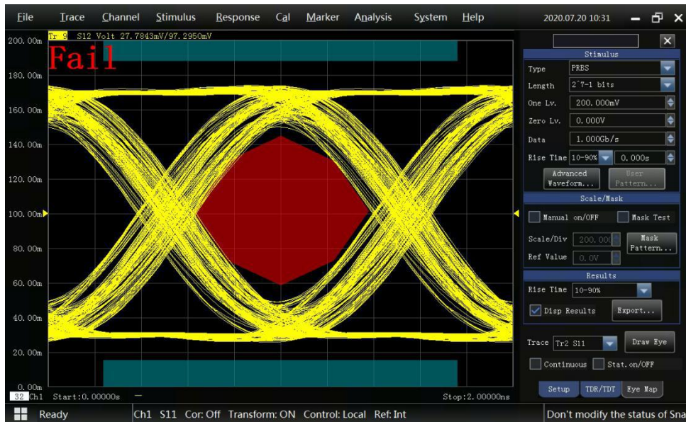
Add Jitter
